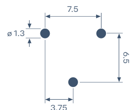
Maßstab 2:1 Scale 2:1
