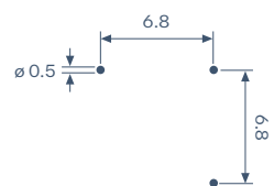
Maßstab 2:1 Scale 2:1
