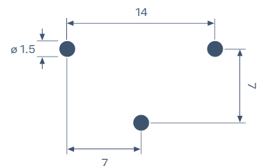
Maßstab 2:1 Scale 2:1
