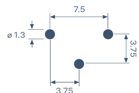
Maßstab 2:1 Scale 2:1
