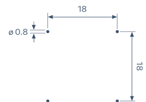
Maßstab 1:1 Scale 1:1
