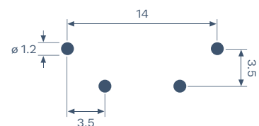
Maßstab 2:1 Scale 2:1
