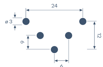
Maßstab 1:1 Scale 1:1
