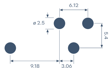
Maßstab 2:1 Scale 2:1
