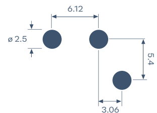
Maßstab 2:1 Scale 2:1
