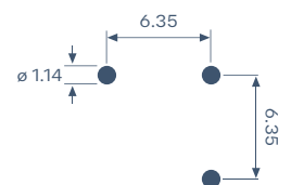
Maßstab 2:1 Scale 2:1
