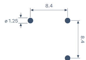
Maßstab 2:1 Scale 2:1
