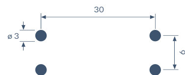
Maßstab 1:1 Scale 1:1
