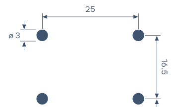
Maßstab 1:1 Scale 1:1
